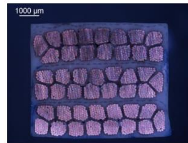
1-MW NASA Motor
