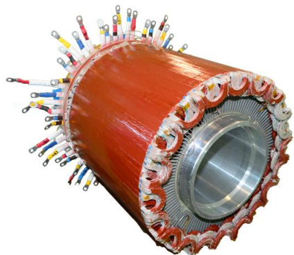
1-MW NASA Motor
